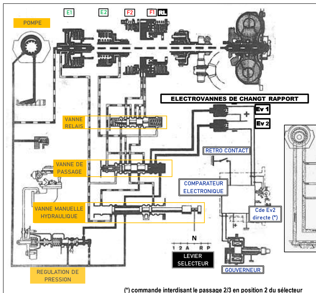
Schéma simplifié
