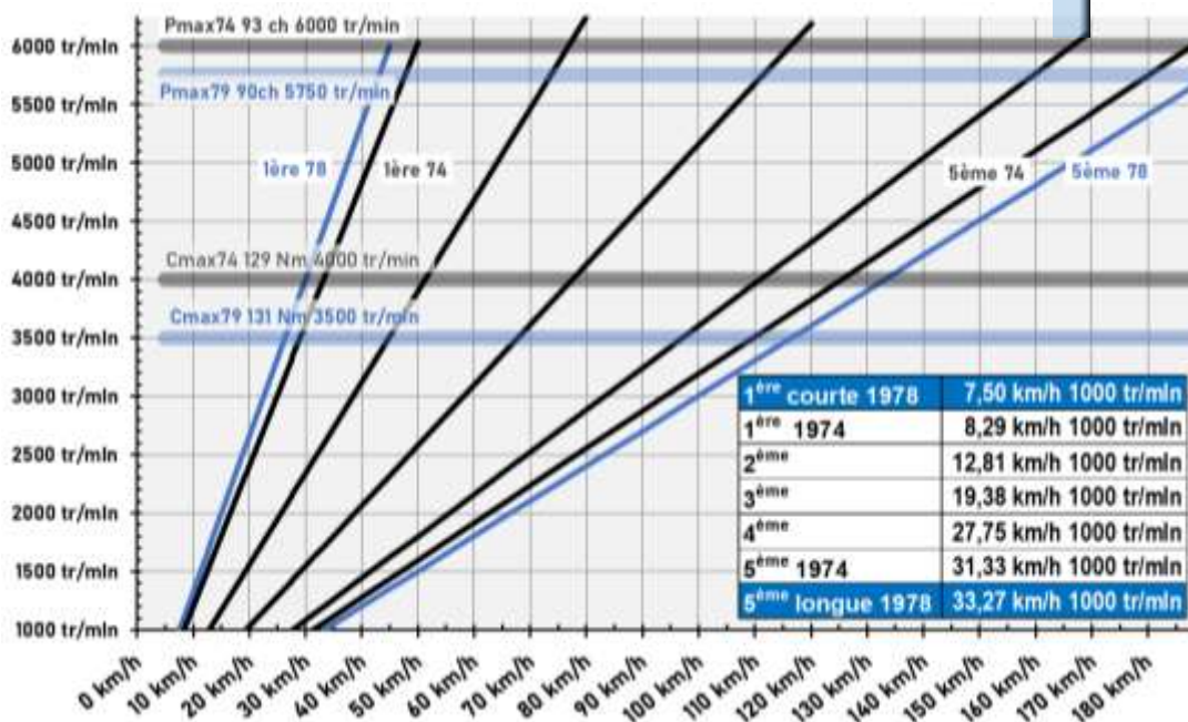
Diagrammes des étagagements TX – BM5 Définitions 1974 et 1978
