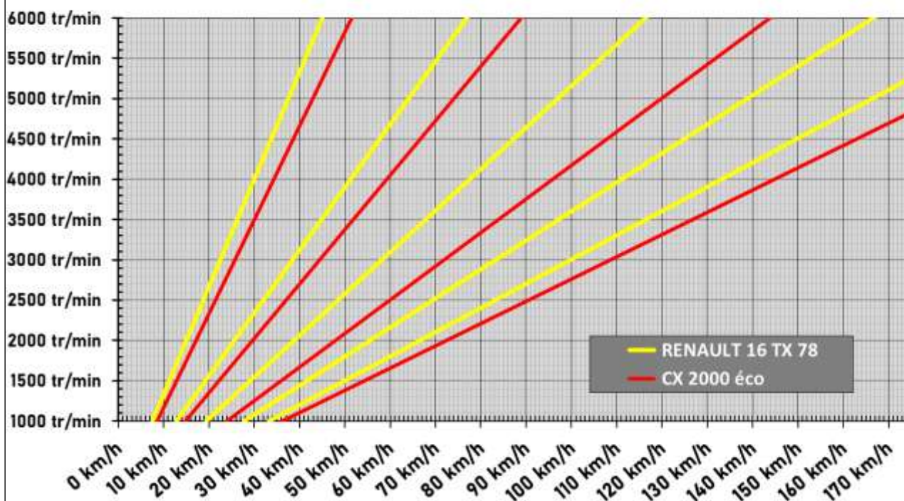
Comparaison des diagrammes CX 2000 éco et RENAULT 16 TX 1978
