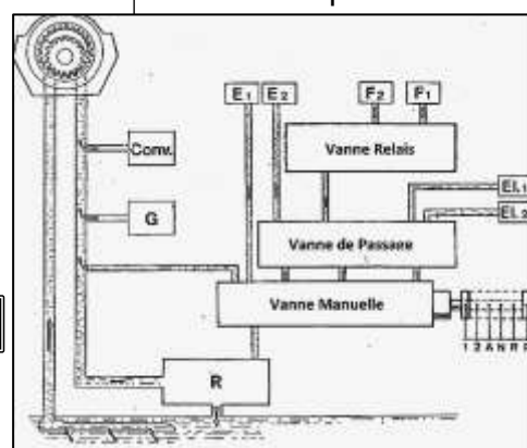
Schéma simplifié
